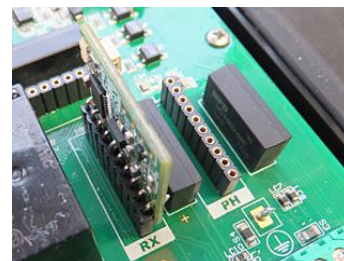
Ranura para el módulo de redox (RX)
